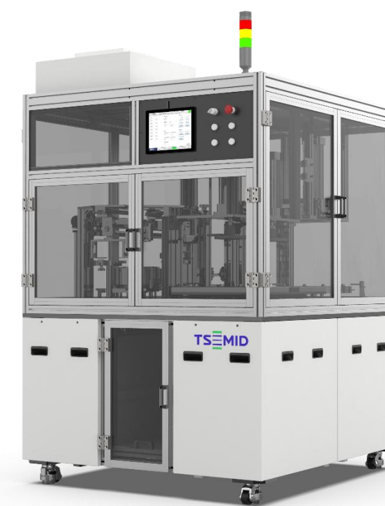
贴蜡机
