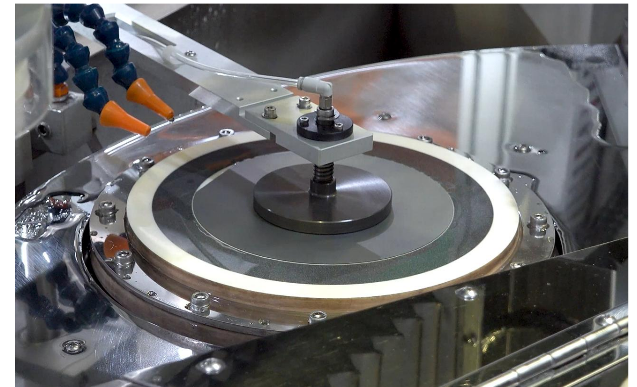
搬运至减薄工位减薄
