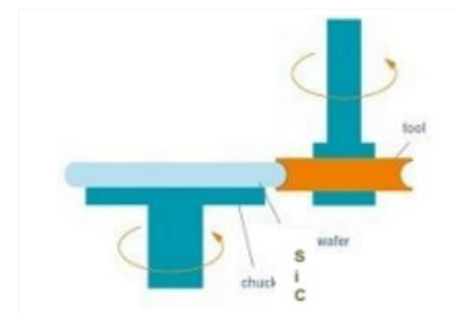
倒边
